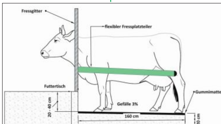
Abb. 3: Flexibler Fressplatzteiler*
