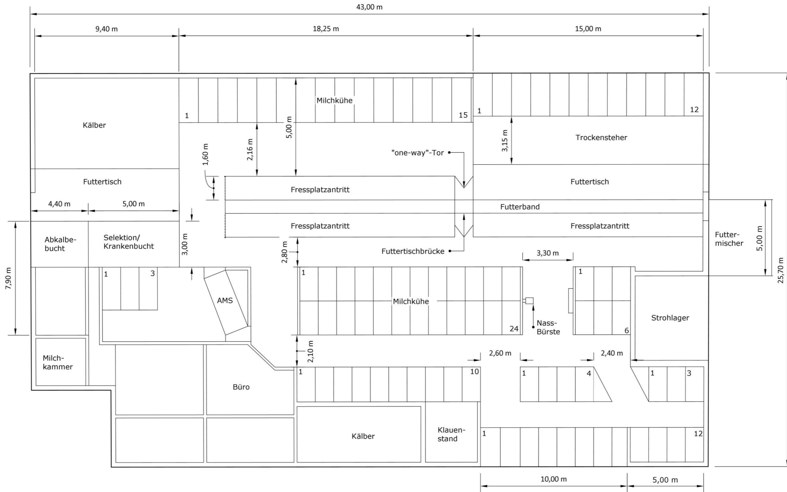
Abb. 12: Grundriss
